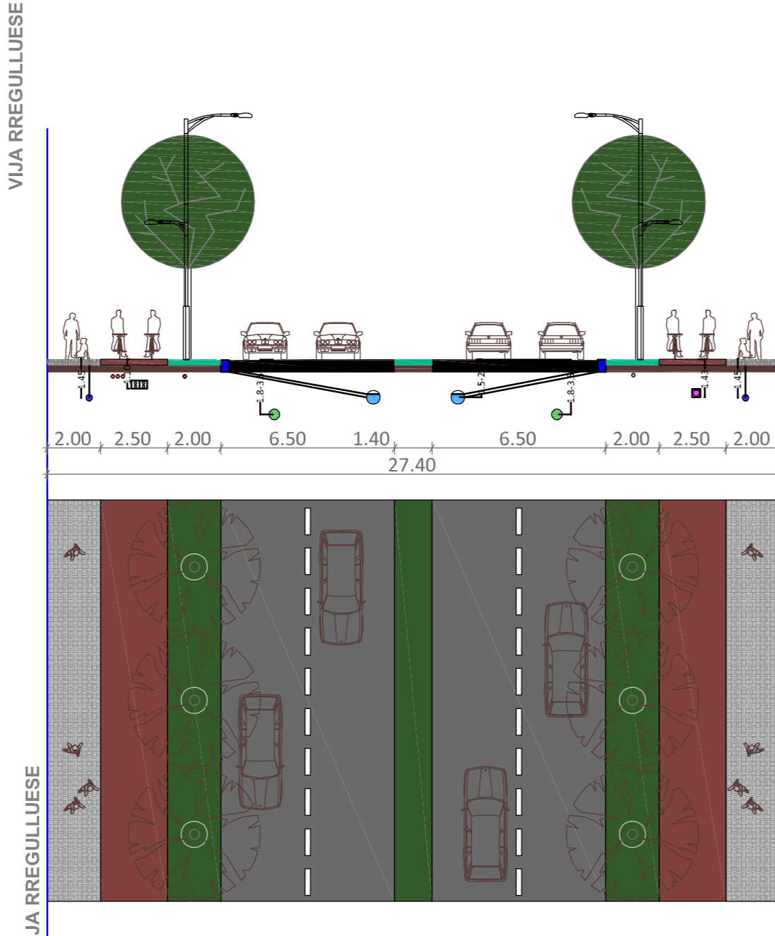
RRUGA QË LIDH UNAZEN E BRENDSHME ME MAGJISTRALEN PRISHTINË-SHKUP (E-E)
