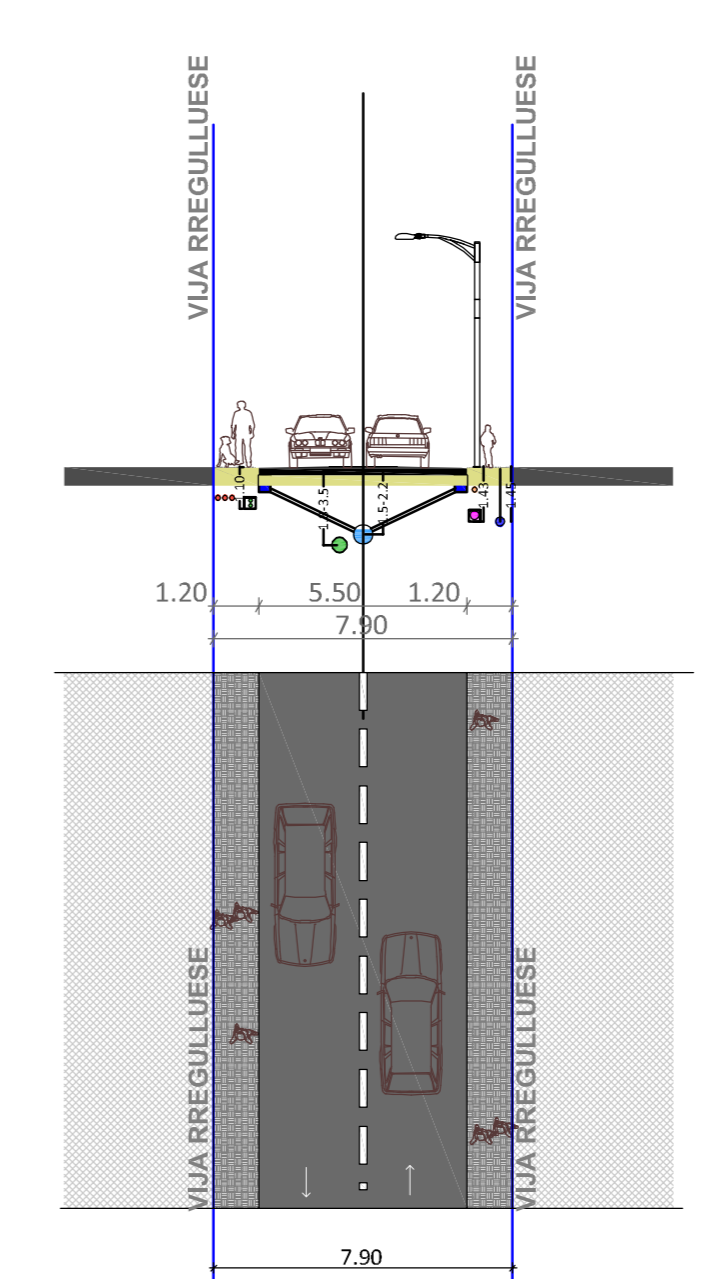
RRUGË PËR QASJE (N-N)
