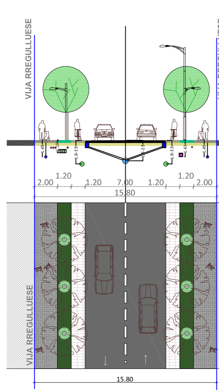
RRUGË LIDHËSE (K-K)
