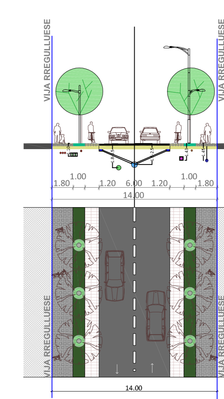
RRUGË LIDHËSE (L-L)
