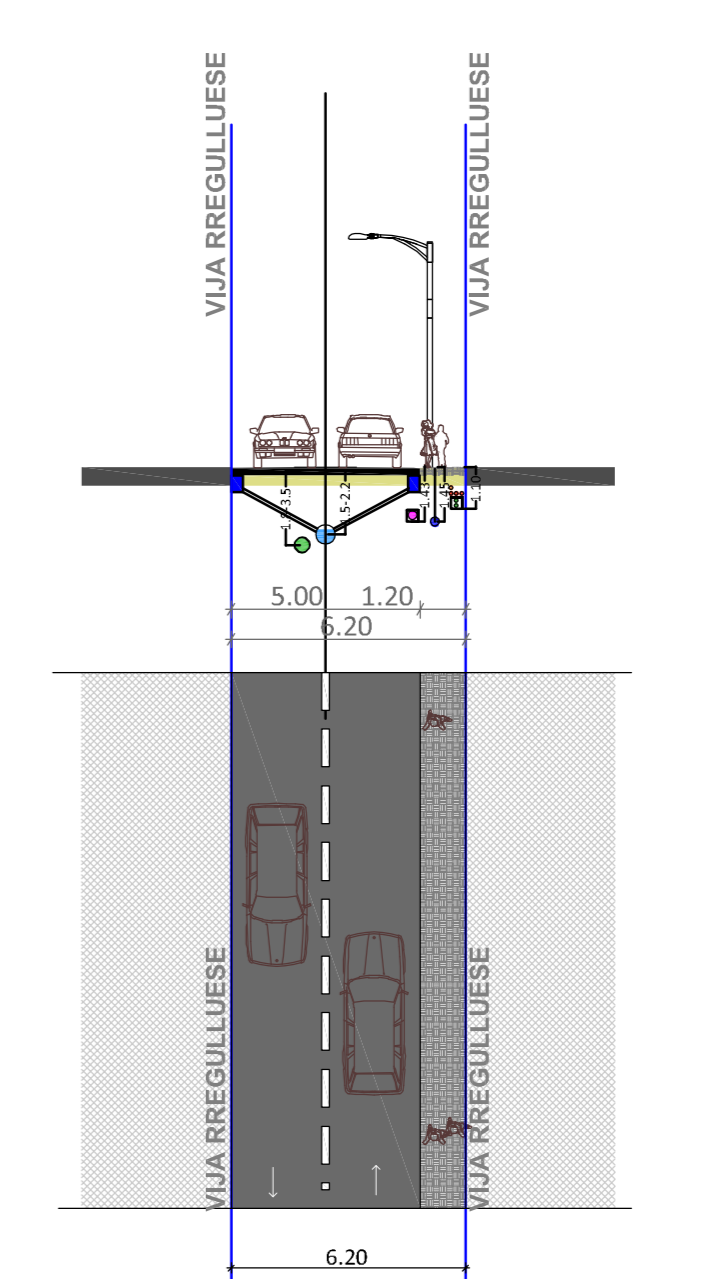
RRUGË PËR QASJE (O-O)
