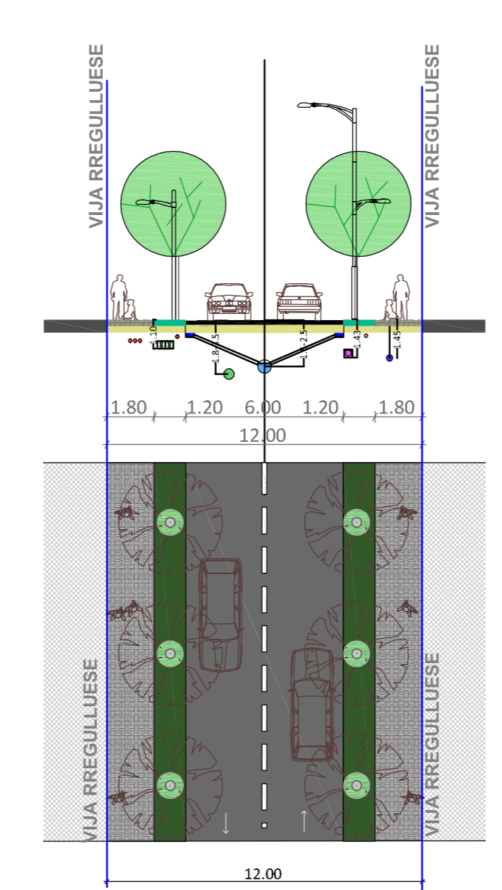
RRUGË PËR QASJE (M-M)
